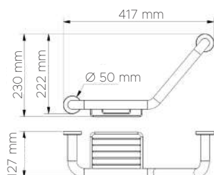
DATOS TÉCNICOS DATI TECNICI 05098
