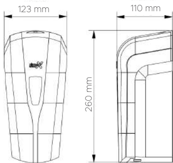
DATOS TÉCNICOS DATI TECNICI 04066
