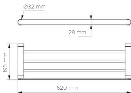
DATOS TÉCNICOS DATI TECNICI 05176
