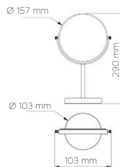
DATOS TÉCNICOS DATI TECNICI 05197
