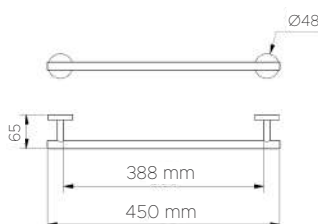
REPISA CON BARRA TOALLERO INFERIOR MENSOLA CON BARRA PORTASCIUGAMANI INFERIORE
