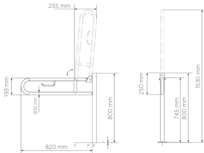
DATOS TÉCNICOS DATI TECNICI 02004 • 02033 • 02110
