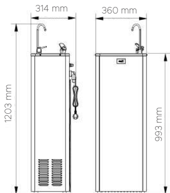
DATOS TÉCNICOS DATI TECNICI 09001
