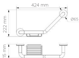
REPISA CON BARRA TOALLERO INFERIOR MENSOLA CON BARRA PORTASCIUGAMANI INFERIORE
