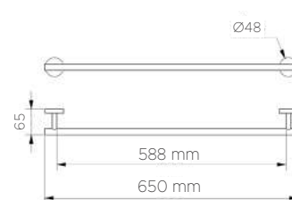
DATOS TÉCNICOS DATI TECNICI 05119 • 05028
