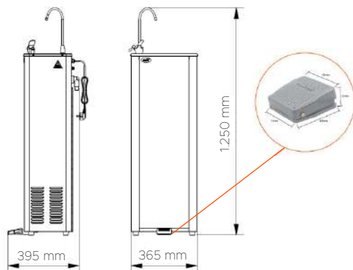
DATOS TÉCNICOS DATI TECNICI 09016
