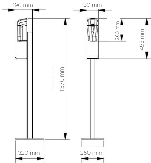
DATOS TÉCNICOS DATI TECNICI 04072
