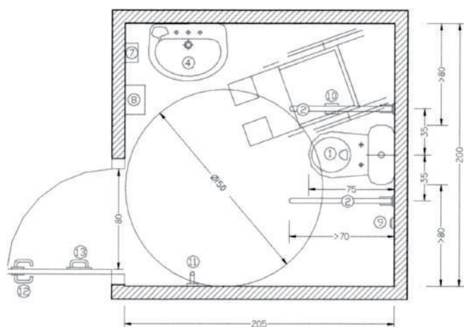
BAÑO ADAPTADO BAGNO ADATTATO
