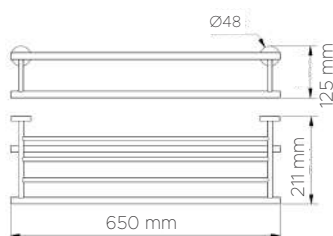
DATOS TÉCNICOS DATI TECNICI 05132 • 05029
