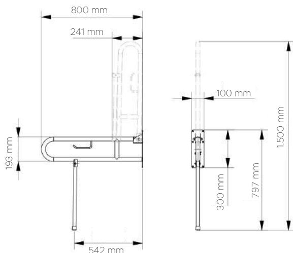
DATOS TÉCNICOS DATI TECNICI 02275 • 02276 • 02281 • 02282
