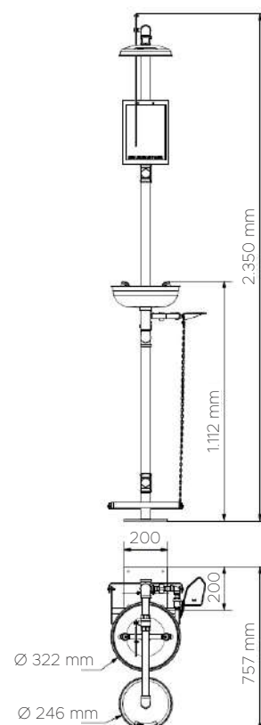
DATOS TÉCNICOS DATI TECNICI 12028
