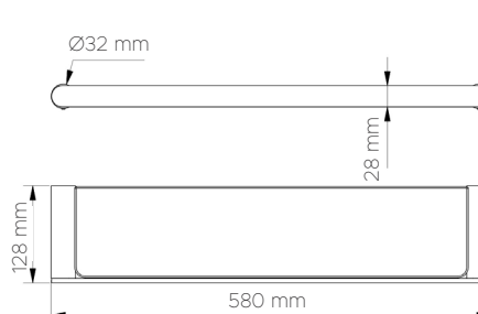
DATOS TÉCNICOS DATI TECNICI 05180
