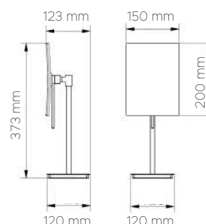
DATOS TÉCNICOS DATI TECNICI 05165
