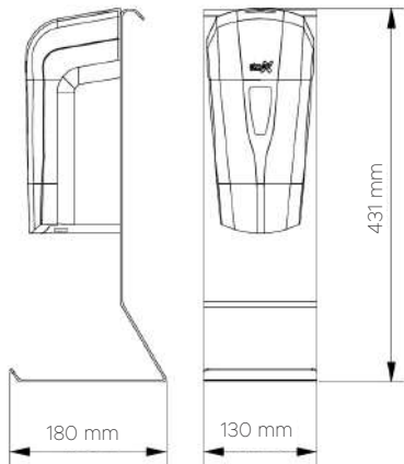
DATOS TÉCNICOS DATI TECNICI 04068
