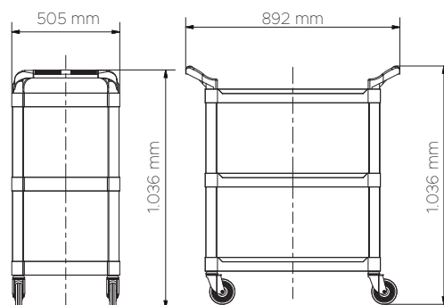
DATOS TÉCNICOS DATI TECNICI 08099
