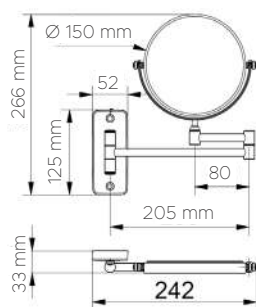
DATOS TÉCNICOS DATI TECNICI 05023
