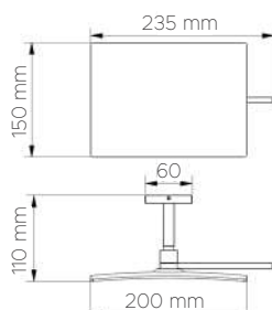
DATOS TÉCNICOS DATI TECNICI 05164
