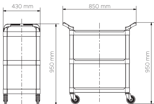
DATOS TÉCNICOS DATI TECNICI 08007
