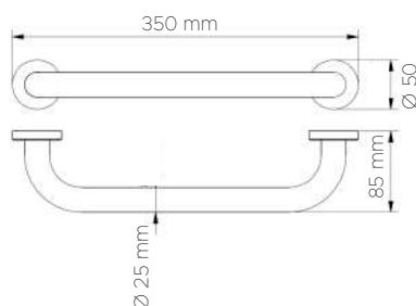
MANILLÓN CON JABONERA MANIGLIONE - PORTASAPONE
