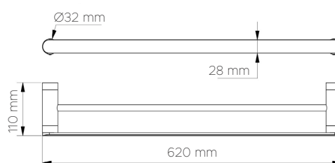
DATOS TÉCNICOS DATI TECNICI 05175
