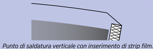
Punto di saldatura verticale con inserimento di strip film.
